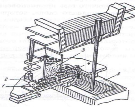
Рисунок 3. Устройство для механической подачи защитной смеси в кристаллизатор [5, 6]: 1 – храповое колесо; 2 – исполнительный механизм; 3 – бункер со смесью; 4 – вал шнека; 5 - кристаллизатор
