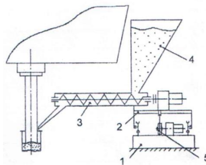
Рисунок 7. Устройство для непрерывной дозированной подачи ШОС в кристаллизатор слябовой машины непрерывного литья заготовок [10]
