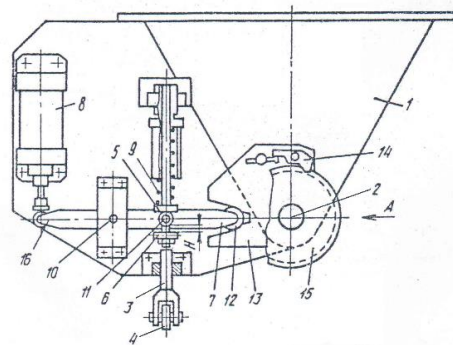
Рисунок 5. Устройство для подачи порошкообразных материалов в качающийся кристаллизатор [8]: 1- бункер; 2- шнековый питатель; 3- штанга-толкатель; 4- ролик; 5 и 6- упоры; 7- двулучий рычаг; 8- пневмоцилиндр; 9- пружина; 10- ось; 11 и 12- ролики; 13- коромысло; 14- собачка; 15- храповое колесо; 16- ролик
