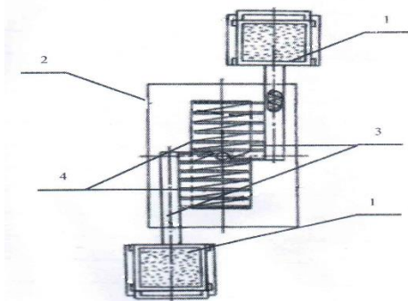
Рисунок 6. Устройство для подачи ШОС в кристаллизатор [9]:
